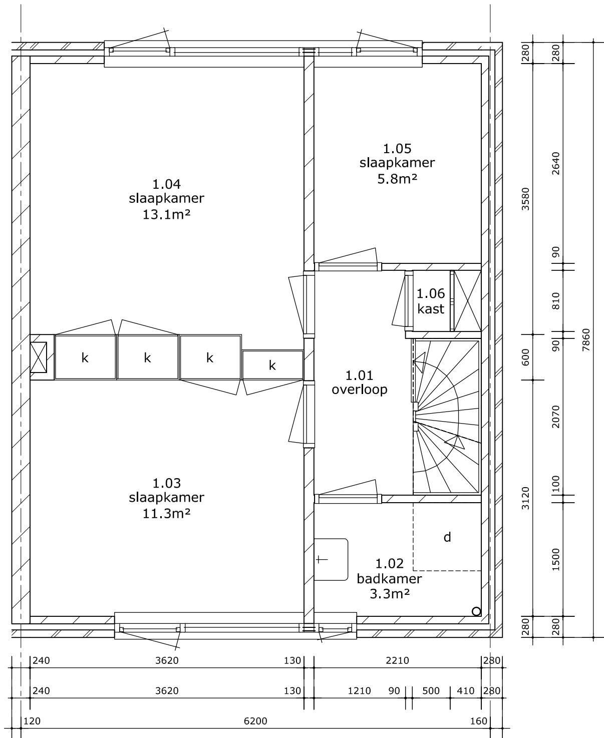
1e verdieping
